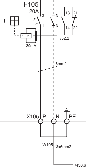
PV-Anlage Wechselrichter 3 (Garagendach)
